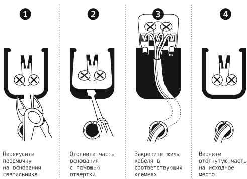
Рис. 3. Порядок монтажа
