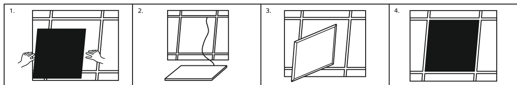
Рис. 3. Порядок монтажа
